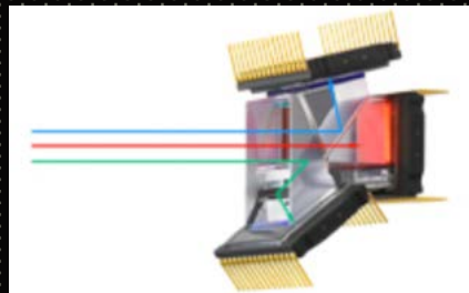
フルカラー3CCDカメラのイメージ
