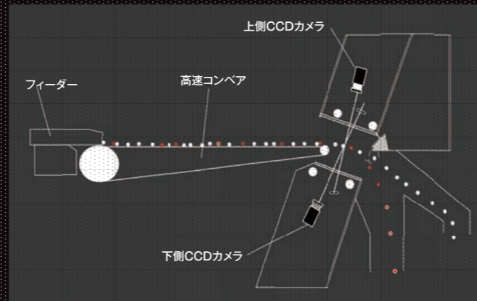
■高速コンベア搬送とカメラによる2方向同時検査 High Speed Conveyor Feeding and 2 side simultaneous inspection by CCD Camera
