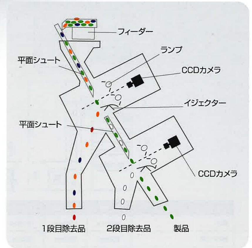
選別の仕組み
